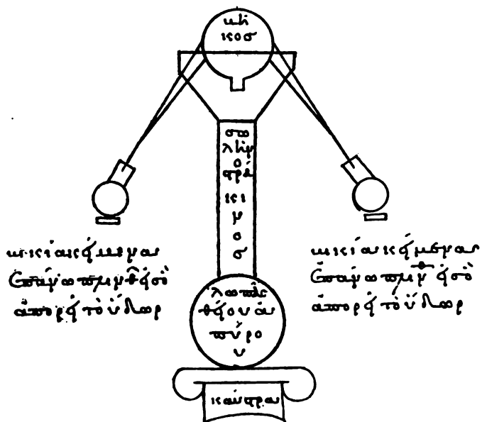
FIGURES 14 et 14 bis. — Alambic à deux réipients ( diibicos ) Réduction aux 2/3.
